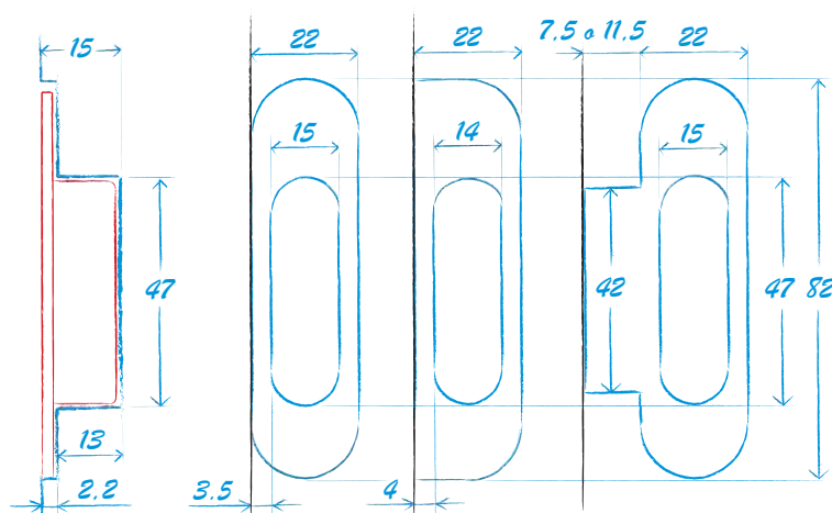
fresate su telaio a battente
