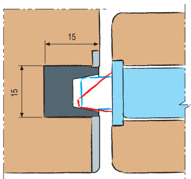
Applicazione su porte a filo con aletta
