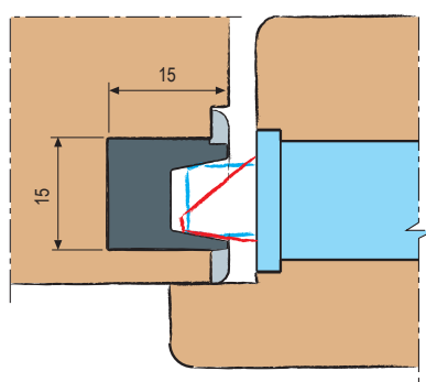
Applicazione su porte a battente
