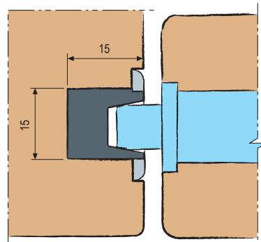
Applicazione su porte a filo senza aletta
