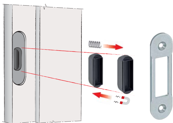
Esempio di fresata su telaio a battente
