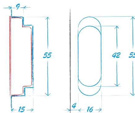
fresata su telaio a battente
