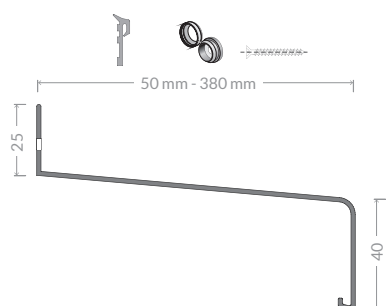
Сечение отлива Classic
