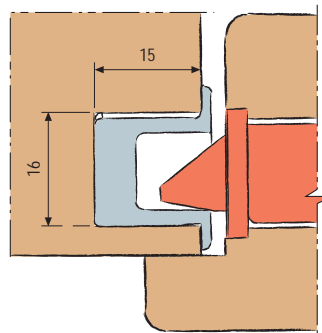
Установка AGB Mediana Polaris в дверь с фальцем
