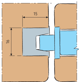
Установка AGB Mediana Polaris в плоскую дверь
