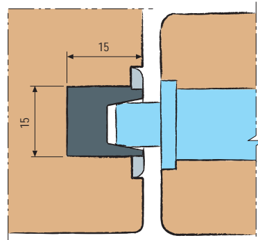
Установка Easy-matic ответной планки на плоскую дверь с замком Mediana Polaris
